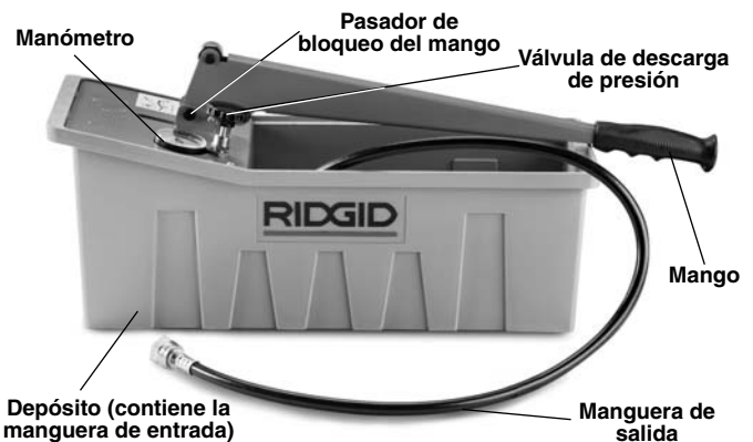
Figura 1 – Bomba 1450 para pruebas de presión
