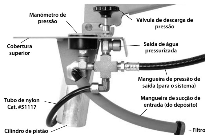
Figura 2 – Componentes da bomba
