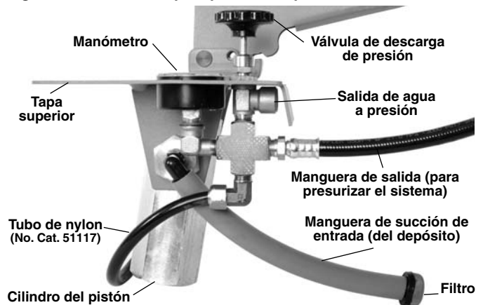
Figura 2 – Componentes de la bomba
