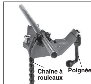
A. Etiau d'établi à chaîne
