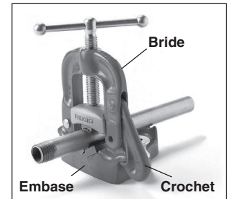
B. Etiau d'établi à bride
