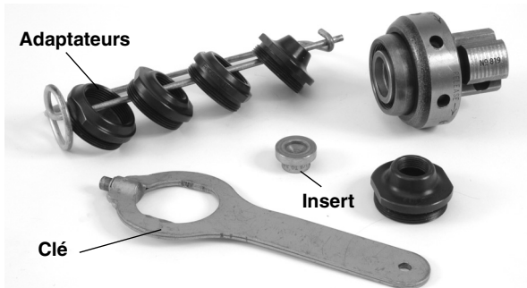
Figure 1 – Mandrin à raccords n° 819 avec accessoires
