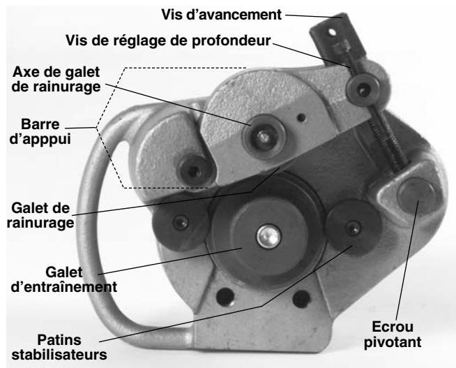
Figure 2 – Séparation des galets de rainurage et d'entraînement
