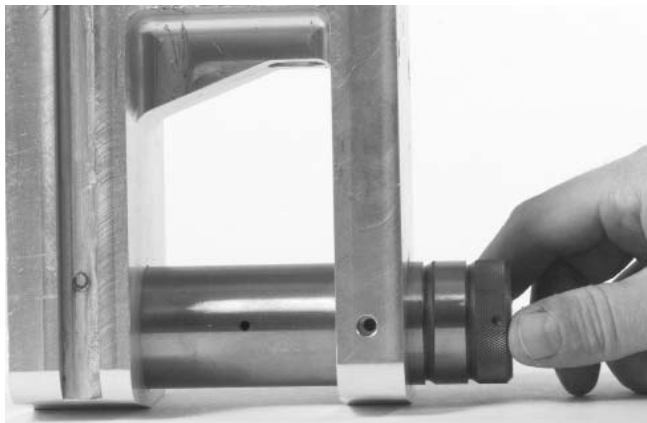
Figura 22 – Alinee el tornillo de retención con la ranura en el árbol
