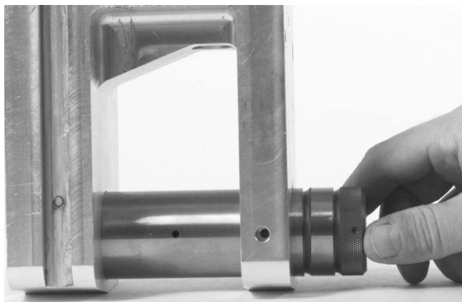
Figure 22 – Alignement de la vis de calage dans la rainure dans l'axe
