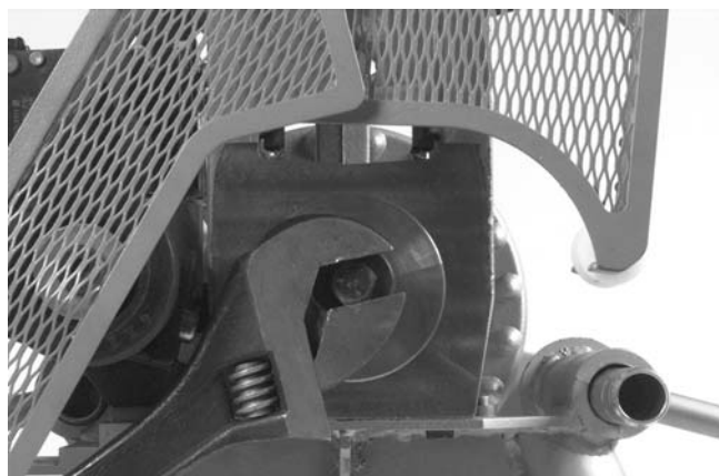
Figure 21 – Desserrage du boulon de serrage de \frac{5}{8} po
