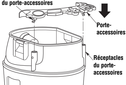
Brides de fixation du porte-accessoires
